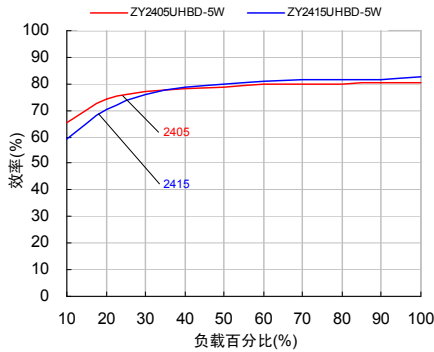
效率与负载关系曲线图
