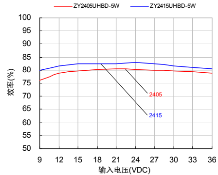
效率与输入电压关系曲线图
