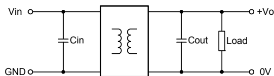
图 1 应用电路图
