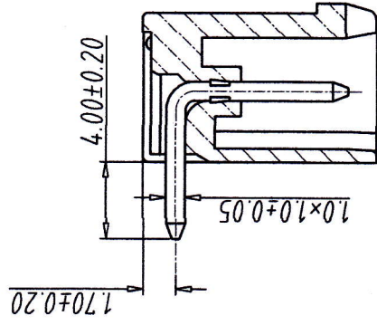
剖面图 A-A
