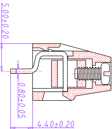
剖面图 A-A
