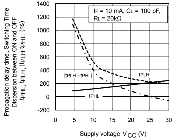
t_{PHL}/t_{PLH}/|t_{PLH}-t_{PHL}| - V_{CC}
