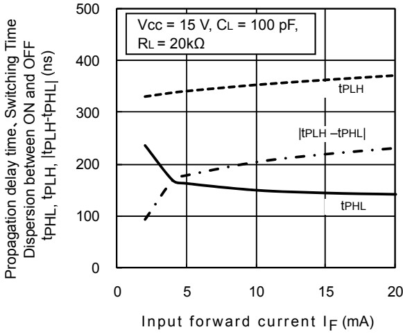
t_{PHL}/t_{PLH}/|t_{PLH}-t_{PHL}| - I_F
