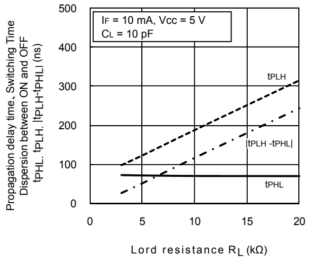
t_{PHL}/t_{PLH}/|t_{PLH}-t_{PHL}| - R_L
