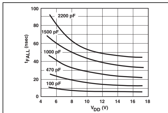
图 2-4: 下降时间-电源电压曲线
