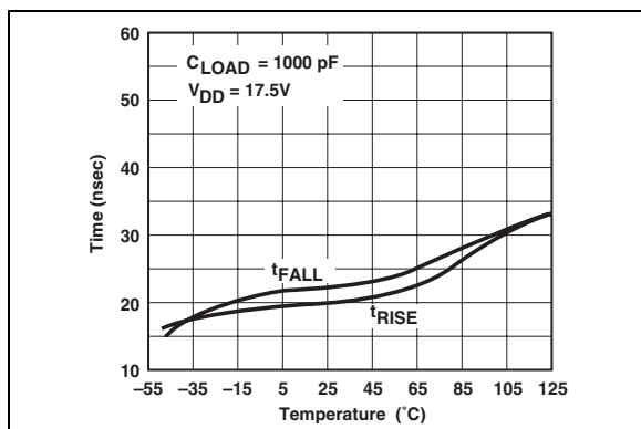
图 2-3: 上升和下降时间-温度曲线
