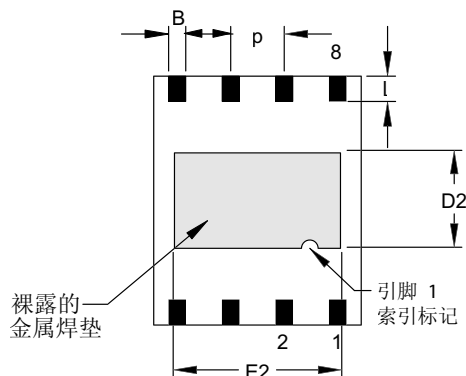
仰视图
