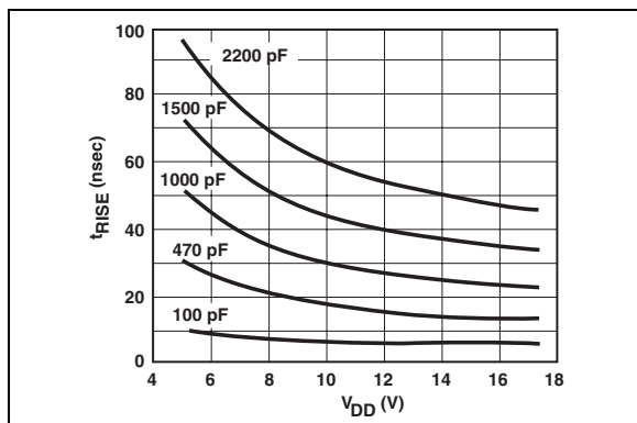
图 2-1: 上升时间-电源电压曲线
