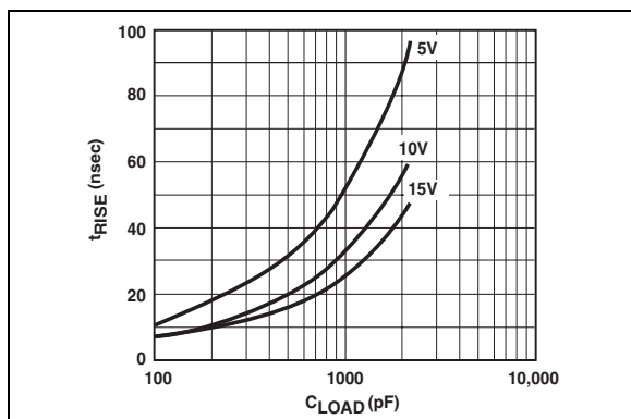
图 2-2: 上升时间-容性负载曲线
