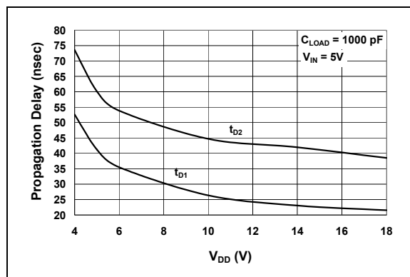
图 2-6: 传输延时-电源电压曲线
