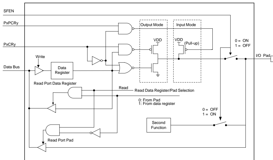
端口模块图
