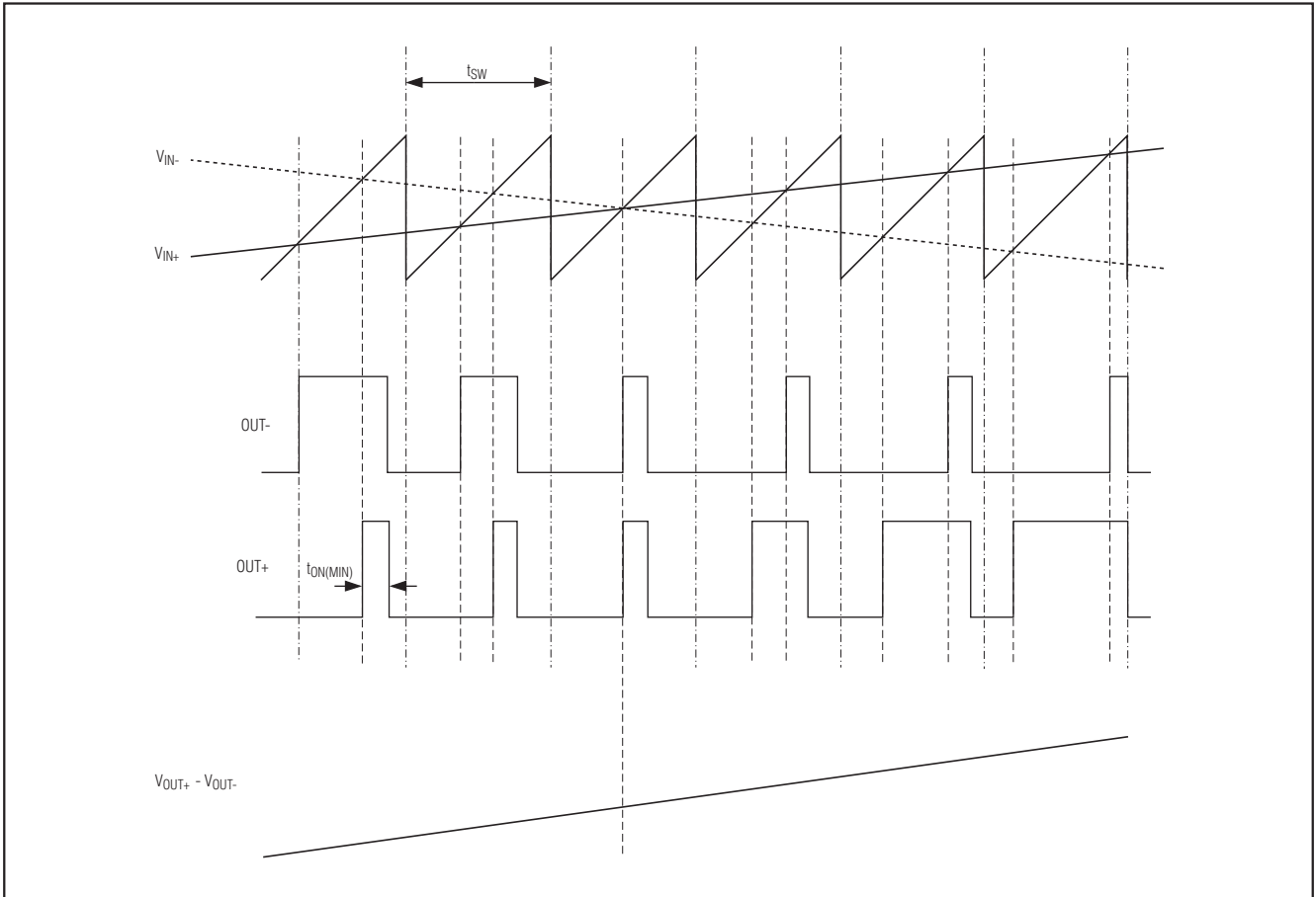
图1. MAX9705输出与输入信号的对应关系
