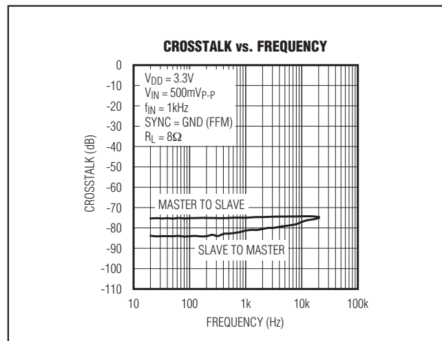
图8. 主-从配置的串扰特性
