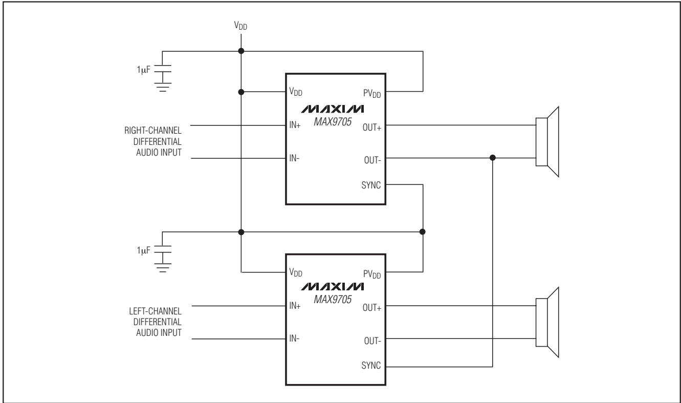
图6. 主-从立体声配置
