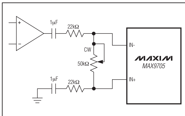
图9b. 改进的MAX9705单端驱动和音量控制
