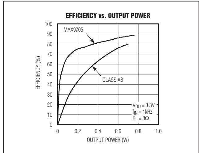
图4. MAX9705的效率与AB类效率的比较
