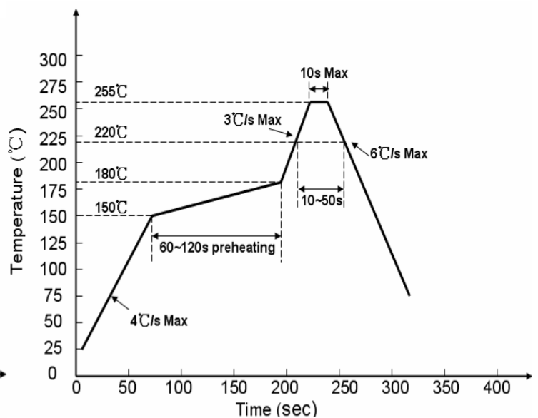
无铅焊接
