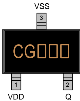
FD2H001BY/SOT23
