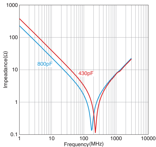
□ 阻抗频率特性
