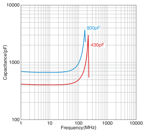
□ 静电容量频率特性
