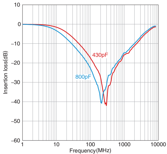
□ 传输特性
