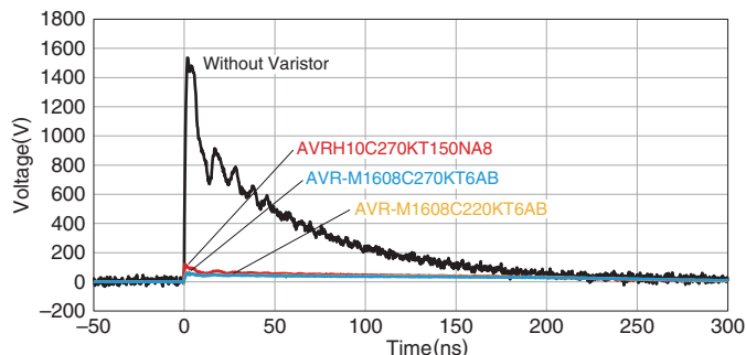
□ 变阻器无, 变阻器设置时的波形
