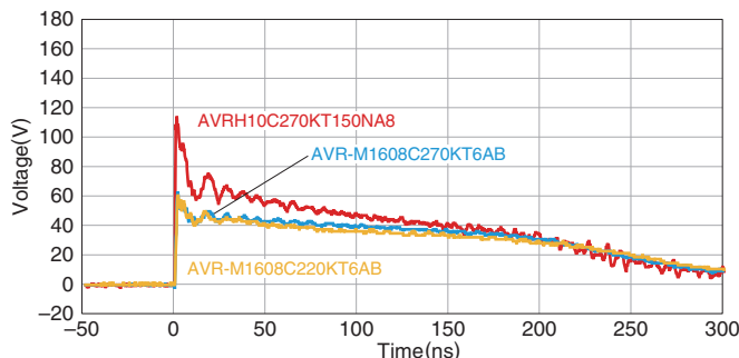
□ 变阻器设置时的波形
