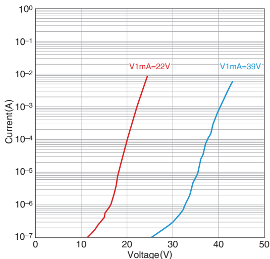
□ 电流-电压特性
