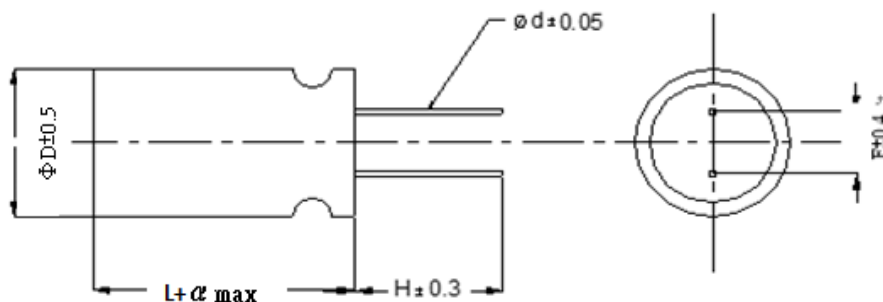
Fig. 2 Dimension
