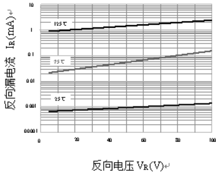
I_R - V_R 关系特性
